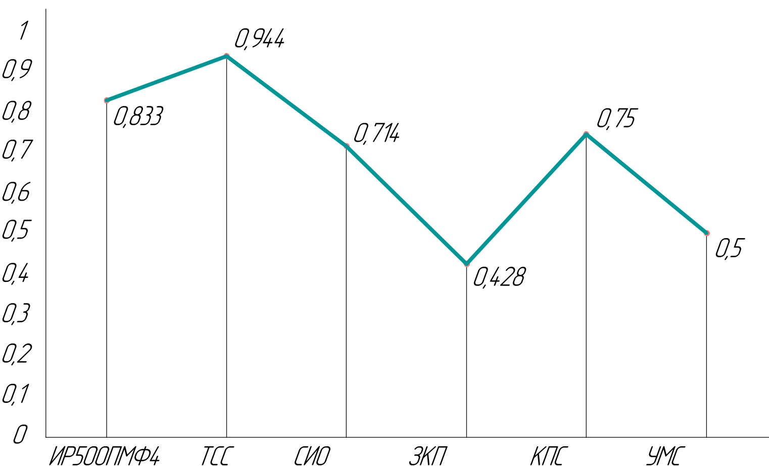
Уровень автоматизации всех систем ГАЗ
